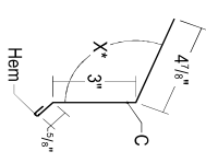
2 Eave Trim 10-2° 55069 / 58069
