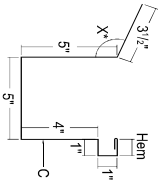
2 Box Gutter 10-2° 55077 / 58077
