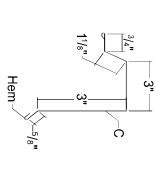
1 Res. Step Rake 10-2° 50023 / 50323
