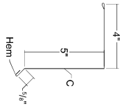
1 Rake Trim 10-2° 55034 / 58034
