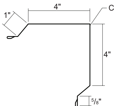
13► ESQUINA EXTERIOR
