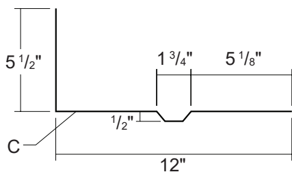
4► SOFITO DE 12"
