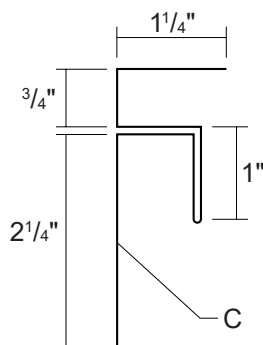
26► CANAL F&amp;J DE 3/4"
