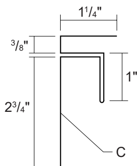
26► CANAL F&amp;J DE 3/8"
