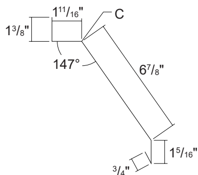
13► ESQUINA EXTERIOR
