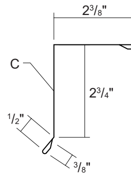
15► MONTANTE DE PUERTA
