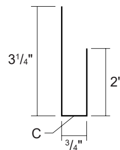
22► ÁNGULO DOBLE
