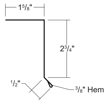
25► MARCO DE ALERO/RASTRILLO
