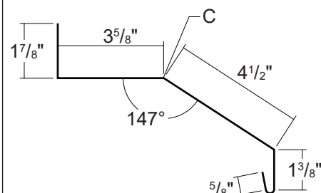
10► CUBIERTA DE RIEL DE MONTAJE SUPERIOR
