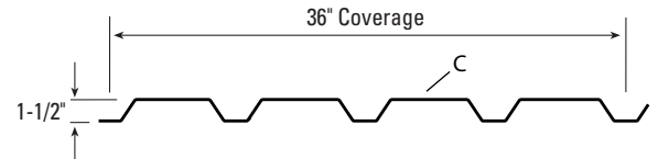
T7-A Wall
